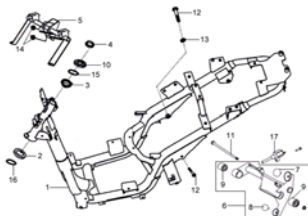
F11 FRAME BODY
