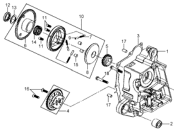
E07 AC GEN. ASSY
