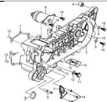
E12 L. CRANK CASE
